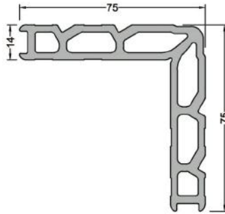
1140 (2,576 kg/mt) L140 KÖŞE TAKOZU 1662
