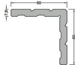
648-3102 (0,805 kg/mt) D48V02 KANAT PROFİLİ 11373
