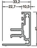
635-1102 (0,788 kg/mt) IP35F02 KASA PROFİLİ 8551
