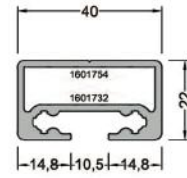
648-3102 (0,805 kg/mt) D48V02 KANAT PROFİLİ 11373
