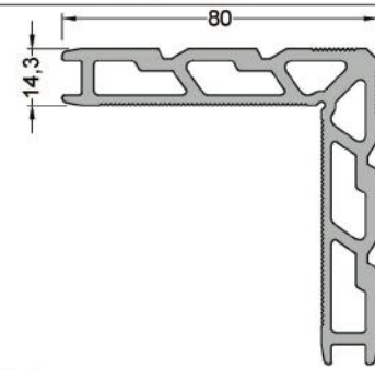
1143 ( 2,867 kg/mt ) L143 KÖŞE TAKOZU
