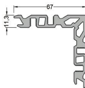
1113 ( 2,188 kg/mt ) L113 KÖŞE TAKOZU
