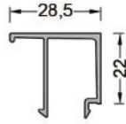
800-285 ( 0,296 kg/mt ) G285 CAMÇİTASI
