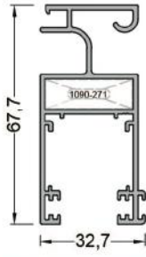
380-4006 ( 1,003 kg/mt ) SLA-S01 SİNEKLİK KANAT PR.
