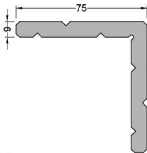
1090 ( 3,284 kg/mt ) L090 KÖŞE TAKOZU
