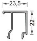
800-235 ( 0,280 kg/mt ) G235 CAMÇİTASI
