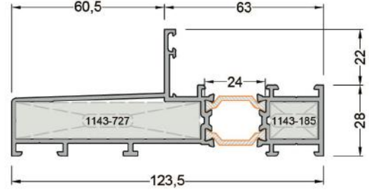
320-1403 ( 1,969 kg/mt ) SAT120F08 SABİT GEÇİŞ KASA PROFİLİ
