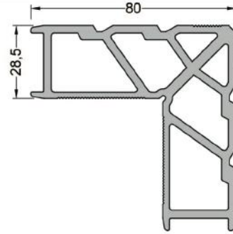
1285 ( 3,511 kg/mt ) L285 KÖŞE TAKOZU
