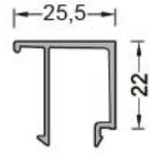
800-255 ( 0,285 kg/mt ) G255 CAMÇİTASI
