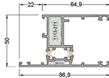
320-2102 ( 1,689 kg/mt ) SAT120V02 SÜRME KANAT PROFİLİ
