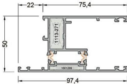
320-2101 ( 1,900 kg/mt ) SAT120V01 KALDIRSÜR KANAT PROFİLİ
