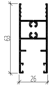
351-2101 (0.867kg/m) KANAT PROFİLİ
