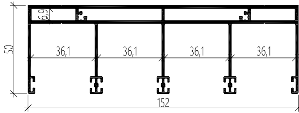
352-1102 (2.679kg/m) ÜST RAY PROFİLİ
