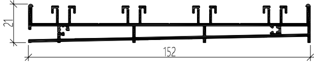
352-1101 (2.011kg/m) ALT RAY PROFİLİ
